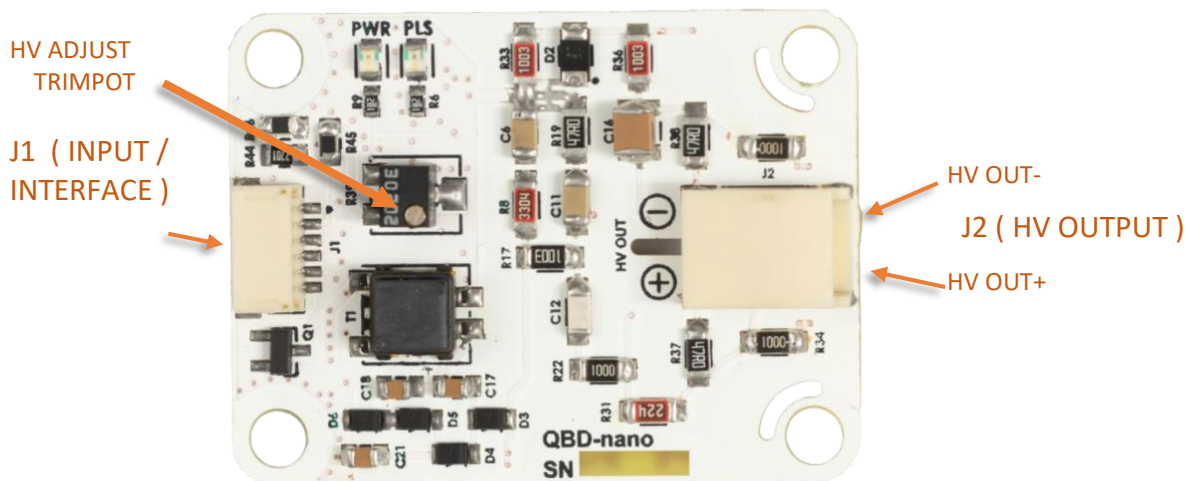
J1 ( INPUT / INTERFACE ) : SM06B-SRSS (JST)
